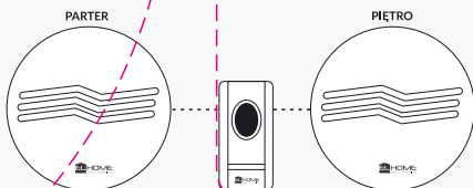
Przykład 2 (dwa dzwonki obsługiwane przez jeden przycisk)
